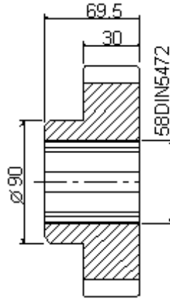
S7/054 Z52 ingranaggio /gear 685
