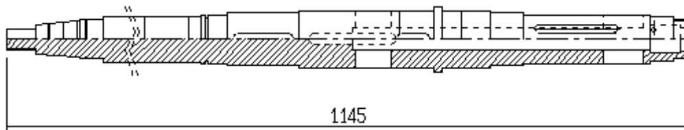
S5/053 Albero portafrizione / clutch-shaft SD50d657d
