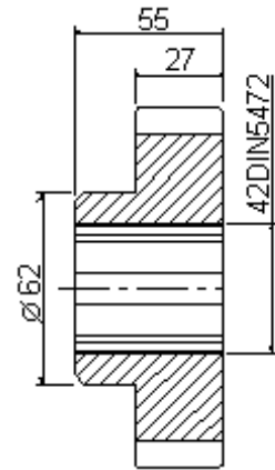
S5/059 Z40 ingranaggio /gear SD50d688b
