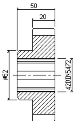
S4/055 Z42 ingranaggio / gear VD25d689
