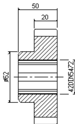
S4/055B Z45 ingranaggio / gear SD25d689
