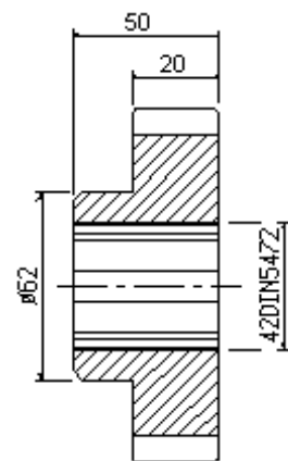
S4/059 Z40 ingranaggio / gear SD25d685
