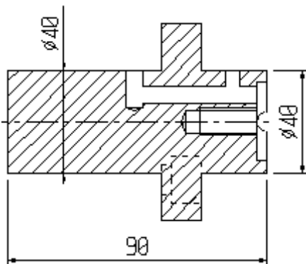
G9/035P perno blocco centrale / centre block pivot
