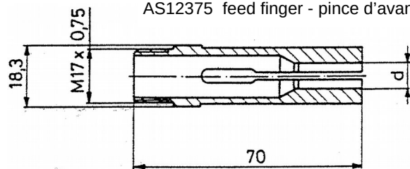
AS12375 feed finger - pince d'avance
