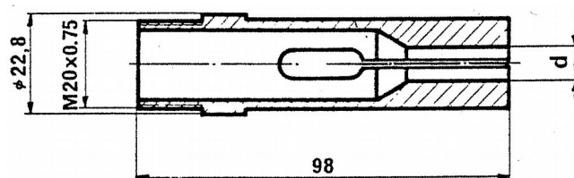
AS12611 feed finger - pince d'avance
