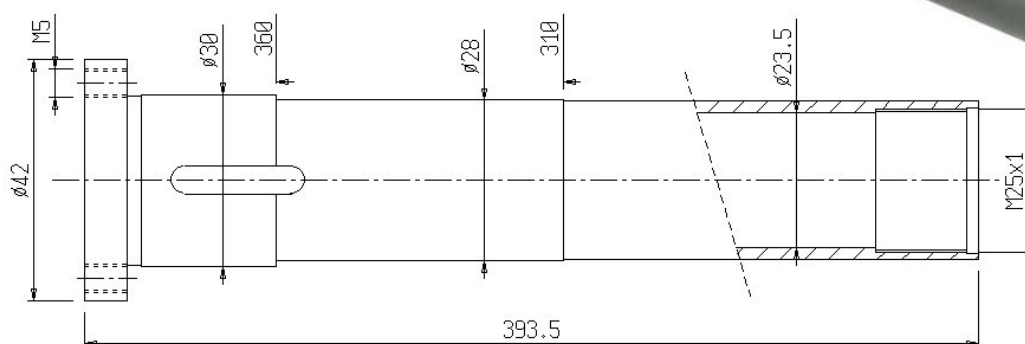
R2/010.6 Collet tube Tube de serrage
