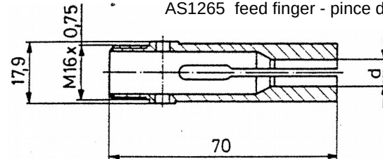
AS1265 feed finger - pince d'avance
